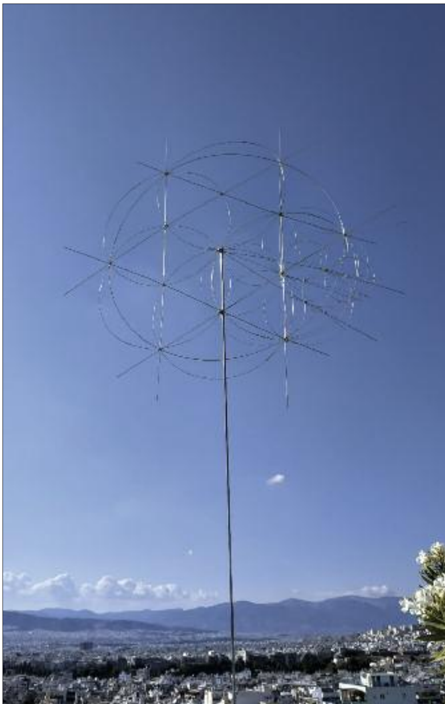
Κυκλισμός-τριχοτόμηση της γωνίας 60^\circ
